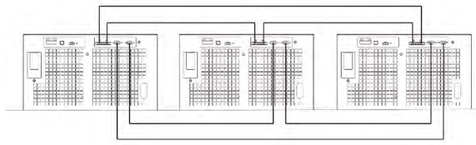
Diagrama 2: Tres SAI en paralelo
