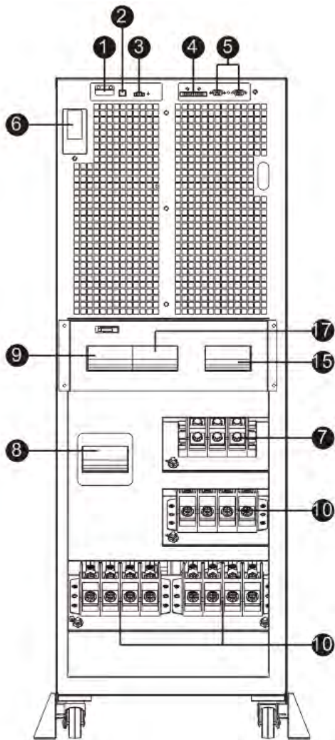
Diagrama 3: 30K Vista frontal con puerta abierta con puerta abierta
